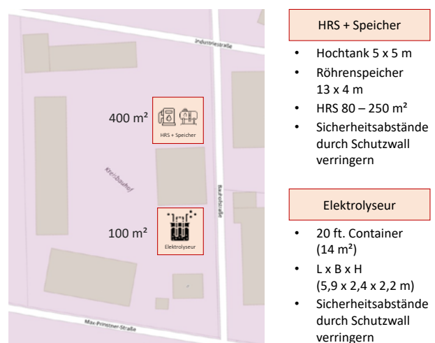
Abbildung 6: Mögliche Verortung der Anlagenkomponenten auf dem Betriebsgelände (Karte: © OpenStreetMap contributors; Grafik von EE ENERGY ENGINEERS GmbH)
